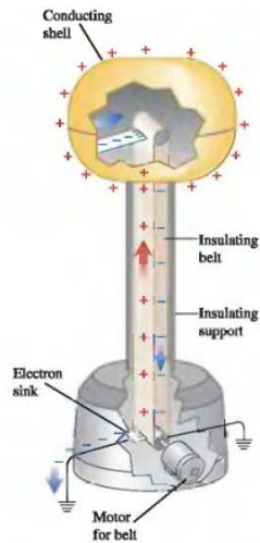
Figura 13. Generador Electrostático de Van De Graaff.
