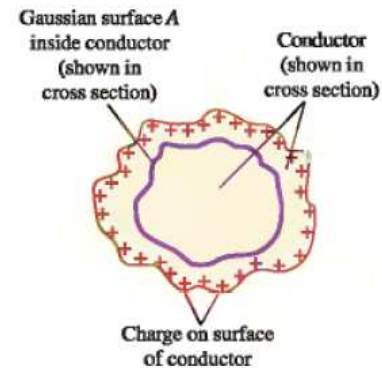
Figura 4. Superficie gaussiana al interior de un conductor.
