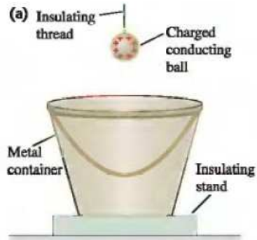
Figura 7. Una pelota conductora cargada con una carga positiva, en presencia de un balde conductor
