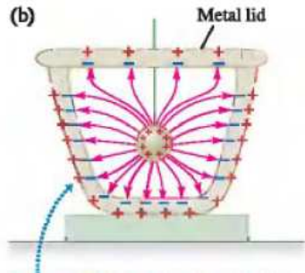
Figura 8. La esfera conductora se baja al interior del balde. Induce sobre él cargas positivas y negativas.
