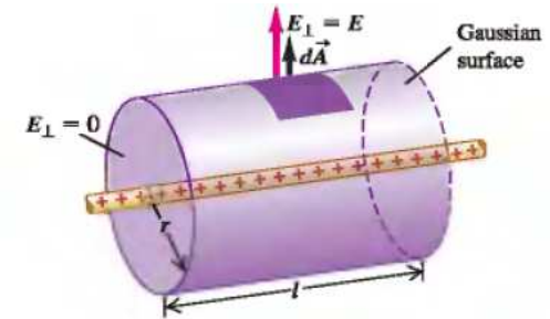
Figura 3. Superficie cilíndrica centrada en el alambre.
