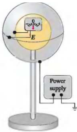
Figura 10. Versión moderna del experimento de Faraday del balde conductor.
