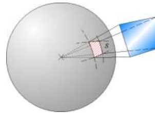
Figura 1. Para calcular el ángulo sólido de un superficie, se proyecta el objeto sobre una esfera de radio conocido R
