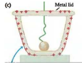
Figura 9. La pelota conductora entra en contacto con la pared interior del balde. Toda su carga se transfiere al balde. Sólo hay carga en la pared exterior del balde
