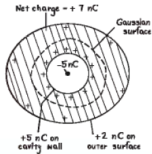
Figura 6. Un conductor sólido con una cavidad tiene una carga total Q . Al interior de la cavidad y aislada del conductor hay una carga puntual q .
