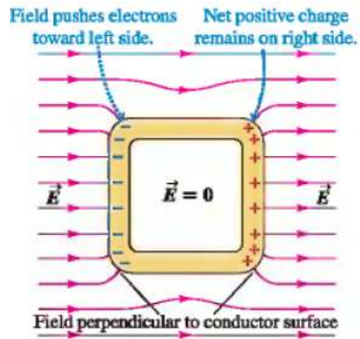
Figura 11. Campo eléctrico creado por una celda de Faraday. El campo eléctrico en la zona interior al conductor se anula.
