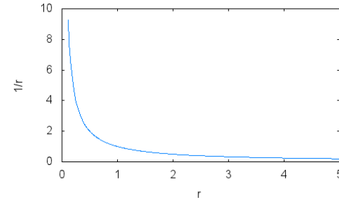
Figura 1. Potencial debido a una carga positiva
