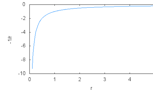
Figura 2. Potencial debido a una carga negativa
